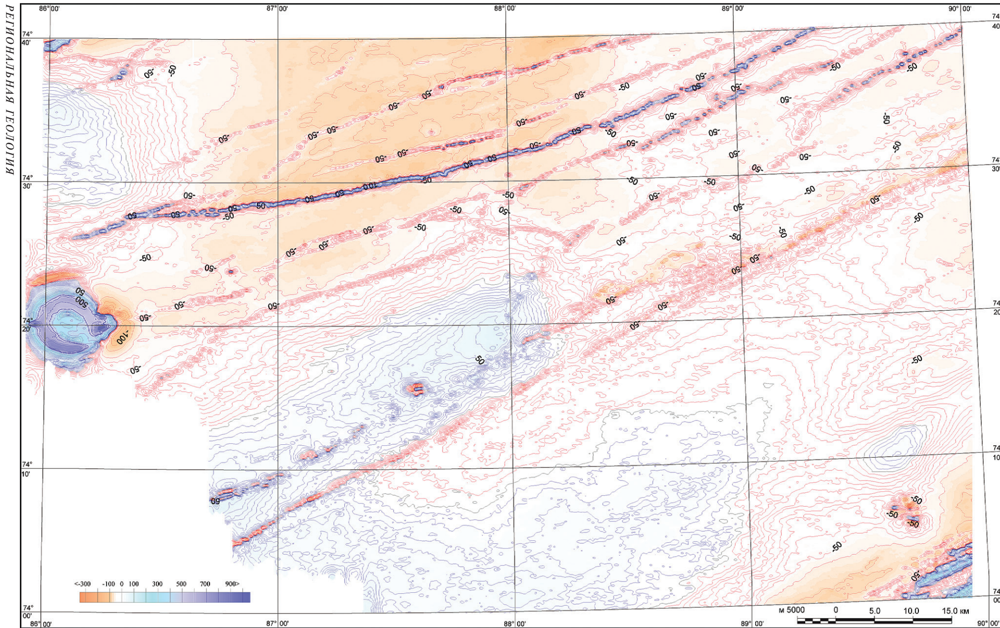
81 Рис. 2. Карта аномального магнитного поля
